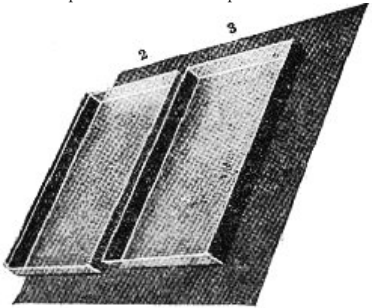
Cage 2 : tôle perforée, force 5/10, dimensions 0,275 x 0,380. Trous de 3mm, à 3mm les uns des autres; les bords sur une largeur de 20mm sont repliés après la coupe des coins. Il n'y a pas de soudure.
