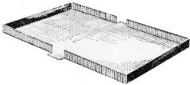
Cage 1 (cage simple) : tôle pleine étamée, force 5/10, dimensions 0,260 x 0,365. Les bords sur la largeur de 20 mm, sont repliés après la coupe des coins. Il n'y a pas de soudure. Une oreille est aménagée sur les deux faces, on la trouve par deux coupes dans les bords repliés.
