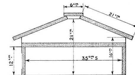
Coupe du toit-chalet
