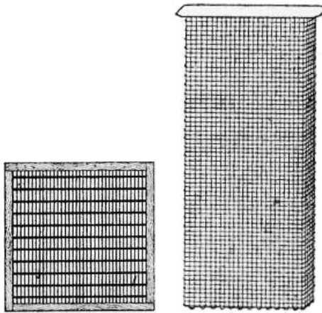
Grille à reine, faite de zinc perforé avec passages de 4,2mm.
